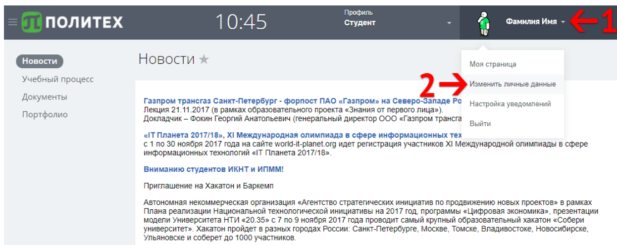
Рисунок 1. Меню пользователя.
